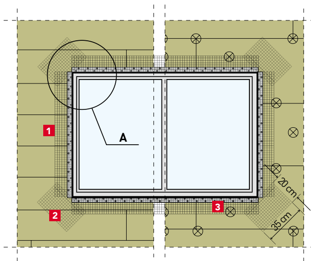
detal A
