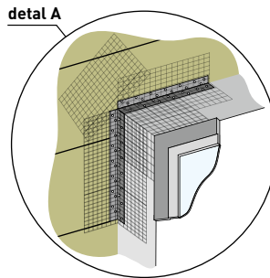
detal A
